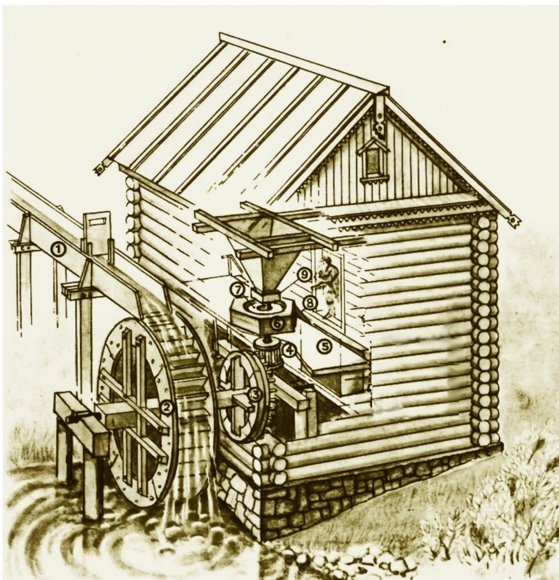
Типовая конструкция водяной мельницы. Именно так был устроен передаточный механизм с водяного колеса на жернова на мельнице в Рудне Шумаровской
